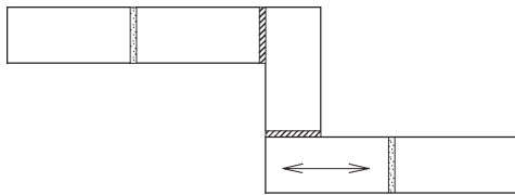
Figura 5: Junta de movimiento vertical por cambio de dirección.
