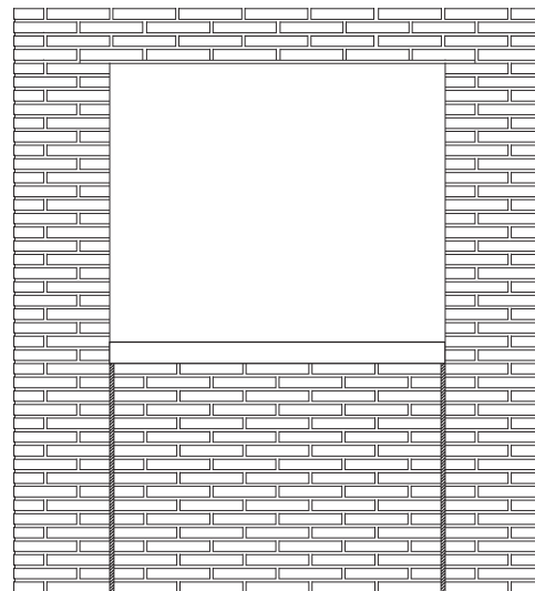
Figura 6: Juntas bajo ventana.
